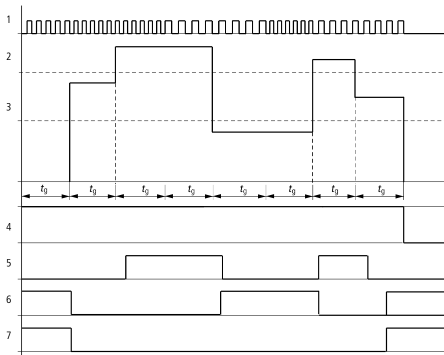
Abb. 145: Wirkdiagramm Frequenzzähler
