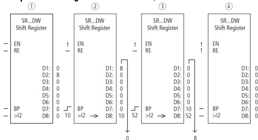
Abb. 187: Schieberegister SR...: Rückwärtsoperation in der Betriebsart DW
