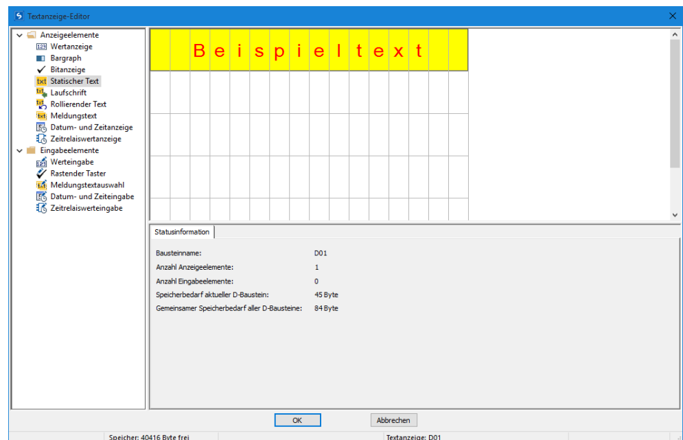
Abb. 195: Textanzeige-Editor mit statischem Text in der ersten Zeile
