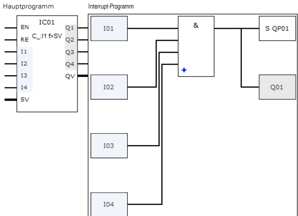
Abb. 208: Übergabe der Zustände von Ein- und Ausgängen zwischen Hauptprogramm und Interrupt-Programm
