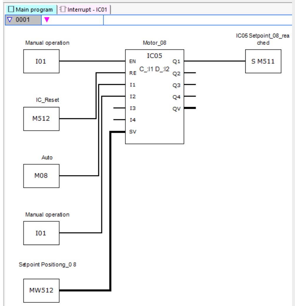
Abb. 213: easySoft 7 Hauptprogramm Inkremental-Wertgeber
