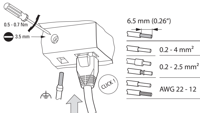
Abb. 33: Ethernet-Leitung anschließen
