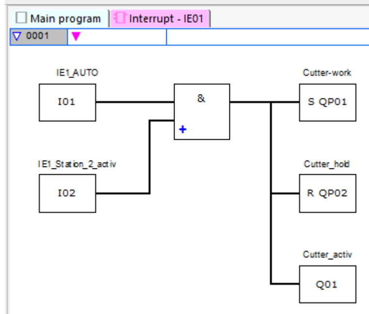
Abb. 219: easySoft 7 Interrupt-Programm Flankengesteuert
