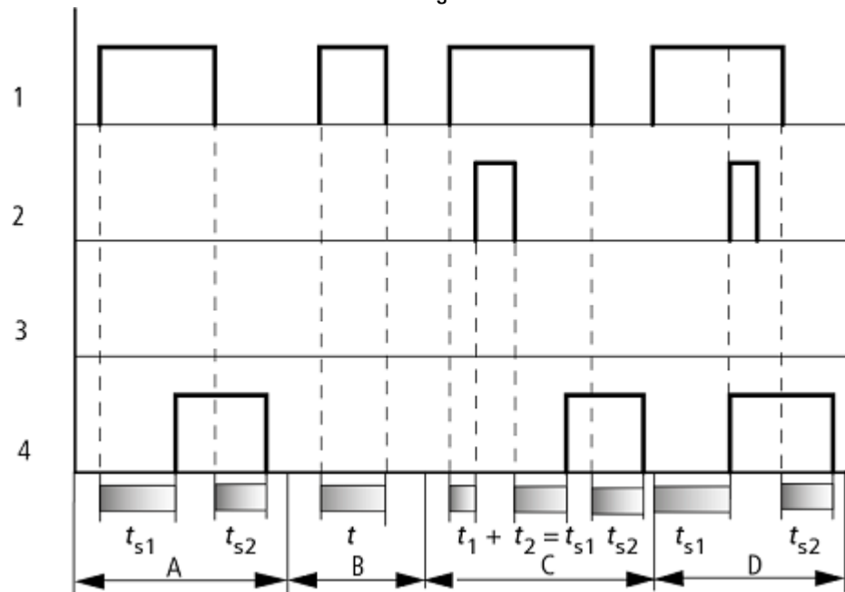
Abb. 122: Wirkdiagramm Zeitrelais, ansprech- und rückfallverzögert 1
