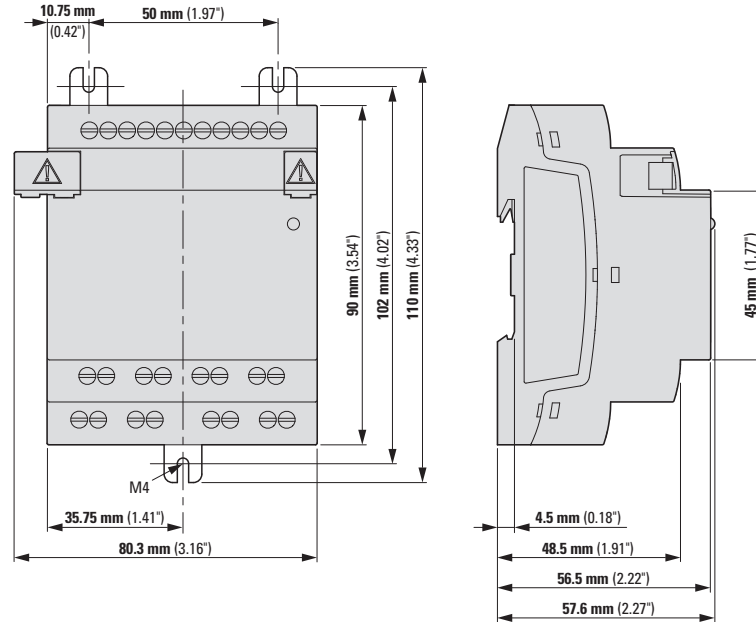
Abb. 296: Abmessungen in mm (Inch) Erweiterungen 4TE
