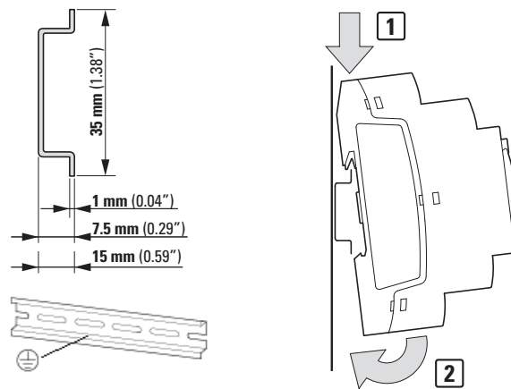
Abb. 7: Montage auf Tragschiene.nach ICE/EN 60715
