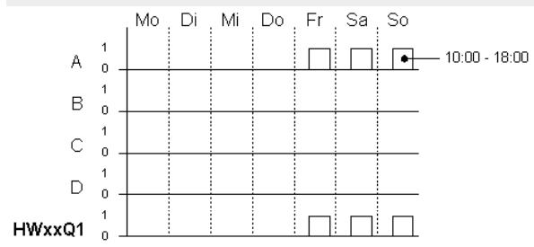
Abb. 99: Wirkdiagramm
