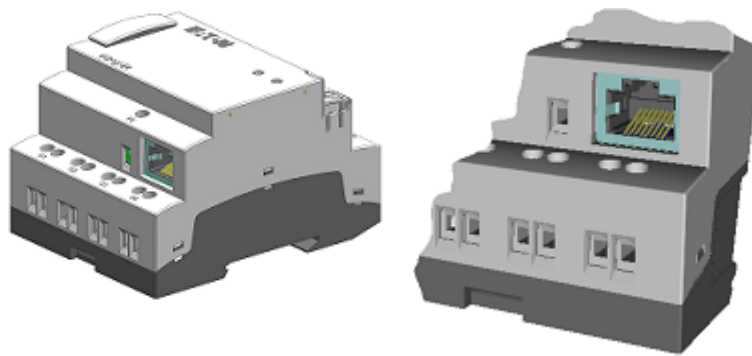
Abb. 29: Ethernet-Buchse am Basisgerät
