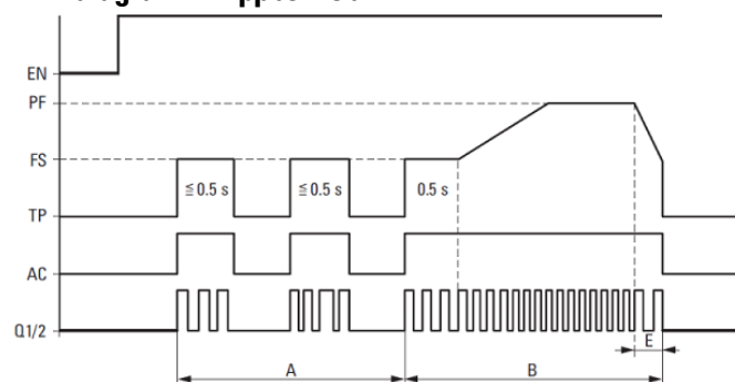
Abb. 169: Wirkdiagramm Impulsausgabe PO - Tipbetrieb
