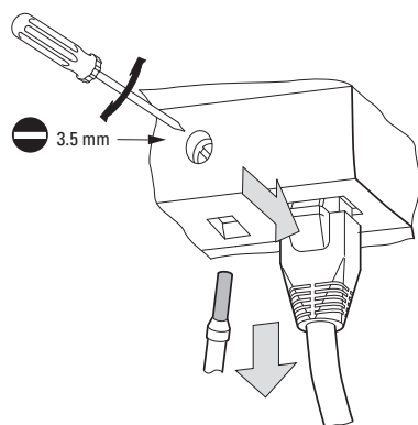
Abb. 34: Ethernet-Leitung entfernen
