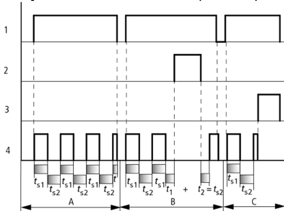
Abb. 125: Wirkdiagramm Zeitrelais, Impulsformend 1
