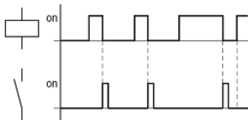
Abb. 80: Wirkdiagramm „Zyklusimpuls“ bei negativer Flanke
