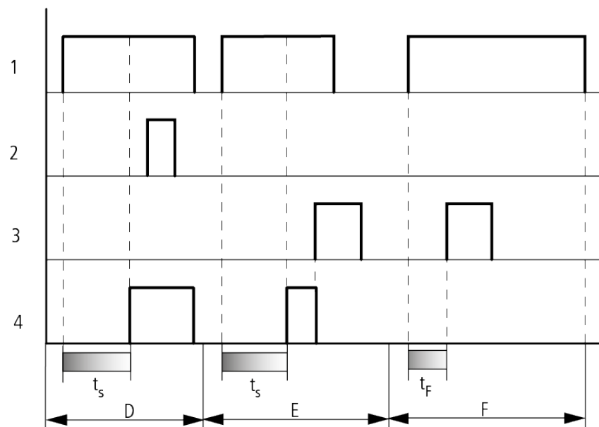
Abb. 119: Wirkdiagramm Zeitrelais ansprechverzögert (mit/ohne Zufallsschalten)
