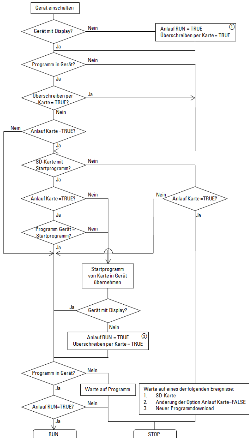
Abb. 55: Einschaltvorgang mit Geräteinitialisierung
