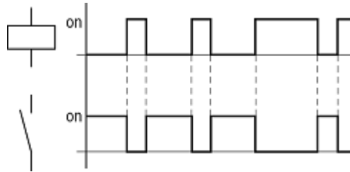
Abb. 78: Wirkdiagramm „inverse Schützfunktion“
