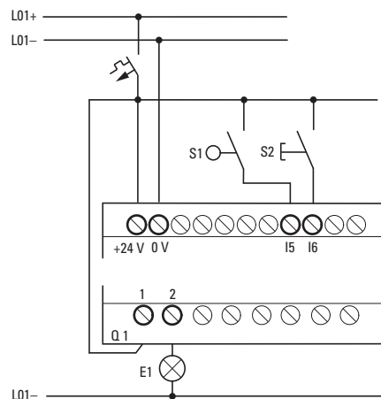
Abb. 238: Verdrahtung z.B. mit EASY-E4-UC...
