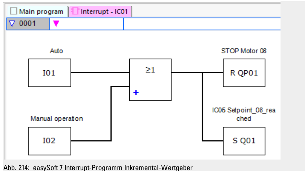
Abb. 214: easySoft 7 Interrupt-Programm Inkremental-Wertgeber
