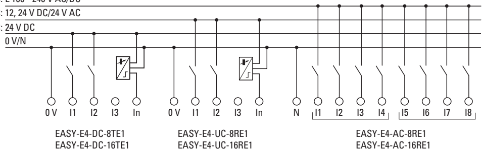
Abb. 16: digitale Eingänge Erweiterungen anschließen
