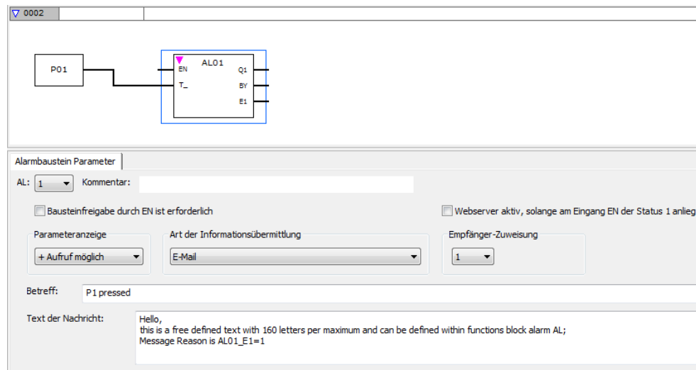
Abb. 293: Register Alarmbaustein mit Parametern des Beispiels und Programm FUP mit Alarmbaustein und P-Taste P01
