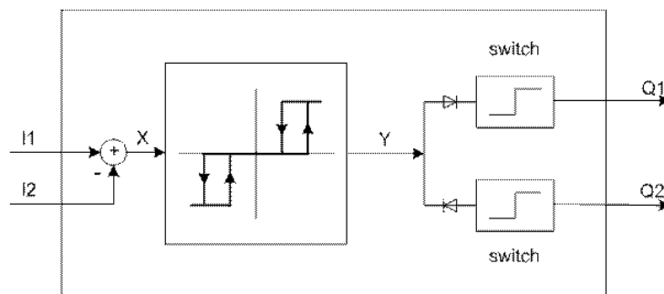
Abb. 172: Prinzipschaltbild Dreipunktregler
