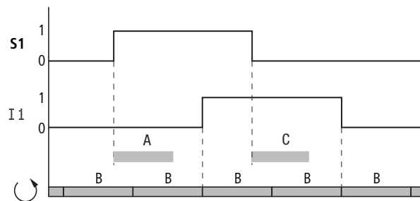
Abb. 258: Verzögerungszeiten bei der Auswertung eines DC-Eingangssignales und aktivierter I-Entprellung
