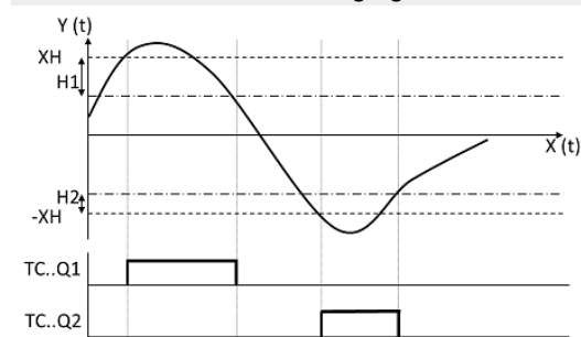
Abb. 174: Wirkdiagramm Dreipunktregler
