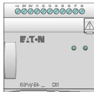
Abb. 49: LED-Anzeige am EASY-E4-...-12...CX1
