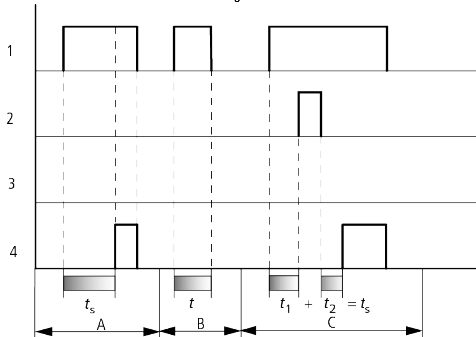
Abb. 118: Wirkdiagramm Zeitrelais ansprechverzögert (mit/ohne Zufallsschalten)
