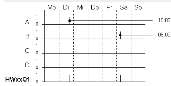
Abb. 103: Wirkdiagramm
