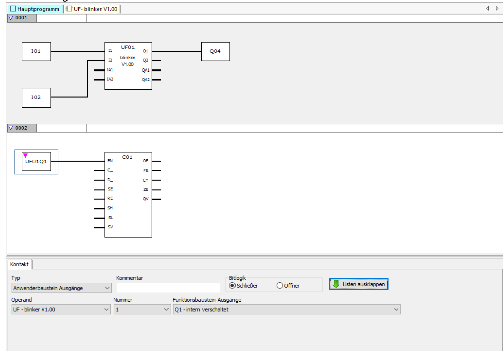
Abb. 228: Ein-/Ausgänge verdrahten
