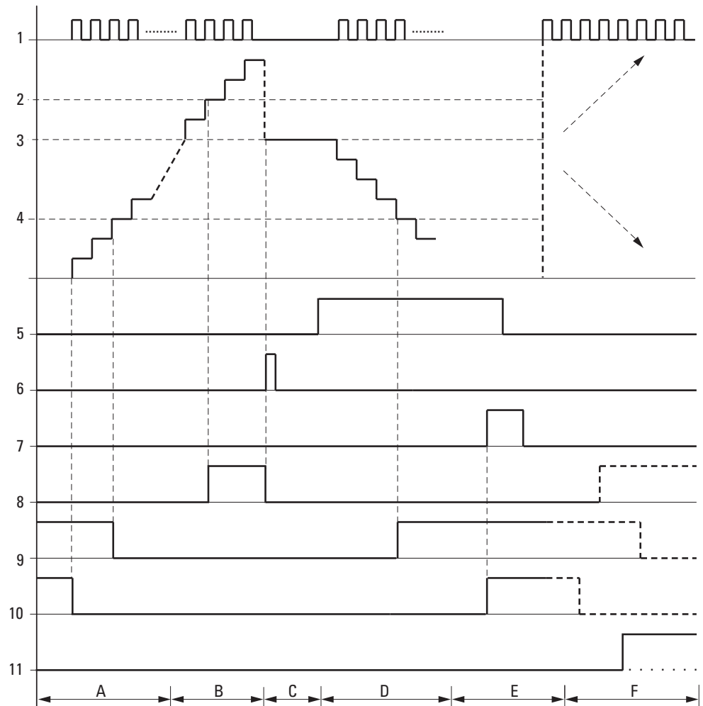
Abb. 146: Wirkdiagramm Hochgeschwindigkeitszähler
