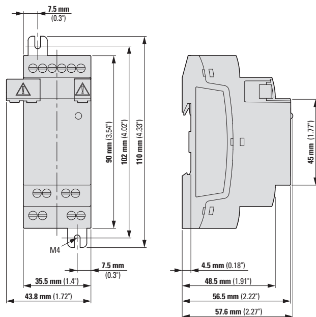
Abb. 297: Abmessungen in mm (Inch) Erweiterungen 2TE
