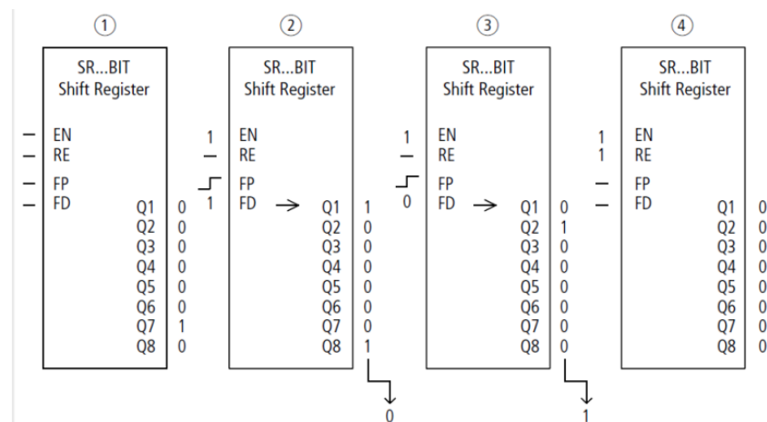
Abb. 186: Schieberegister SR...: Vorwärtsoperation in der Betriebsart BIT
