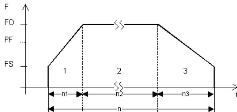
Abb. 170: Typisches Impulsprofil eines Schrittmotors mit den Sequenzen Hochlauf [1], Betrieb [2] und Bremsen [3]
