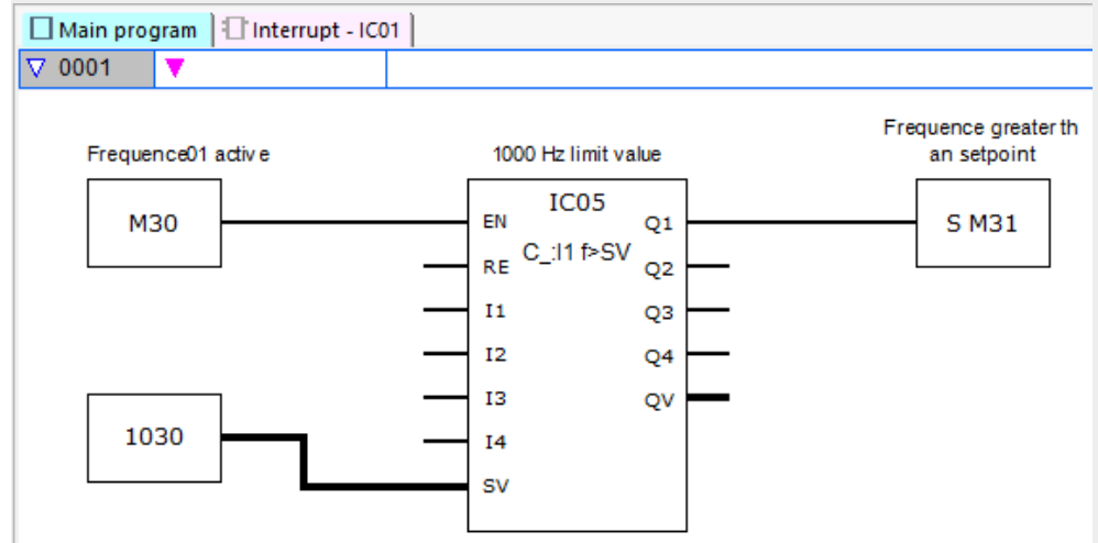
Abb. 215: easySoft 7 Hauptprogramm Frequenzmessung
