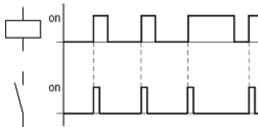
Abb. 79: Wirkdiagramm „Zyklusimpuls“ bei positiver Flanke
