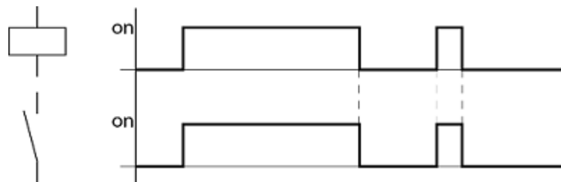
Abb. 74: Wirkdiagramm „Schützfunktion“
