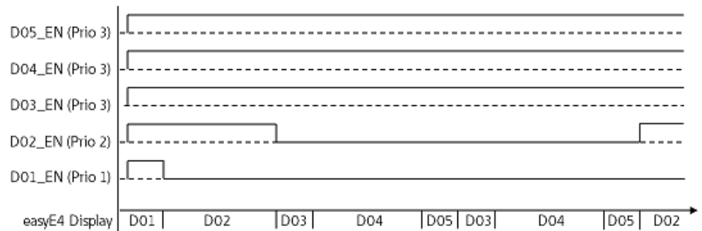
Abb. 194: Wirkdiagramm Textanzeige mit den Textbausteinen gleicher Priorität 3
