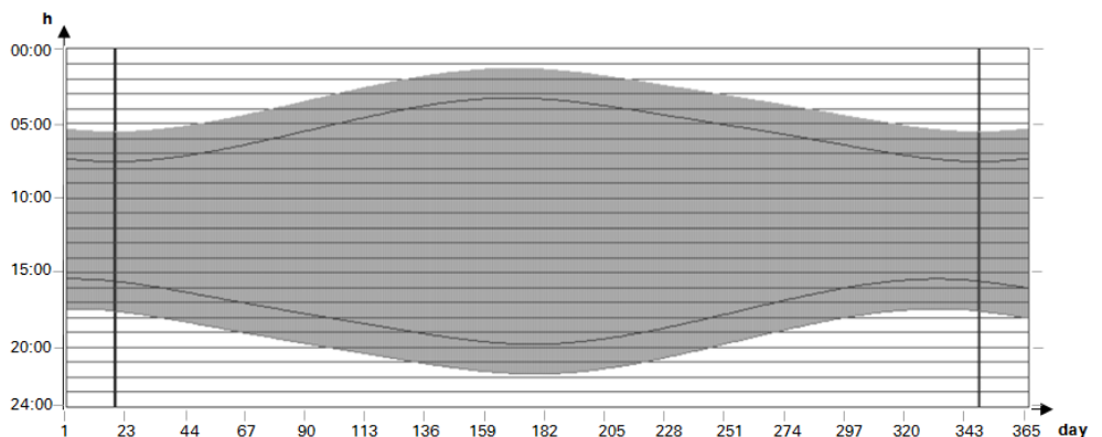
Abb. 140: Offset; O1=-2; O2=2; Q1=1 schaltet 2 Stunden vor Sonnenaufgang ein und 2 Stunden nach Sonnenuntergang aus
