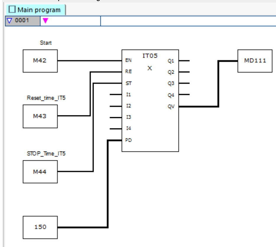
Abb. 221: easySoft 7 Hauptprogramm zeitgesteuert
