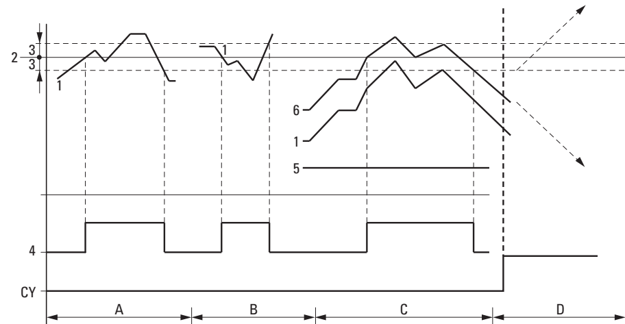
Abb. 150: Wirkiagramm Analogwerte-Vergleicher
