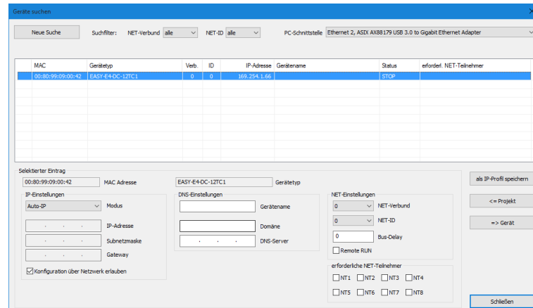
Abb. 267: IP-Profil vom gefundenen Gerät speichern
