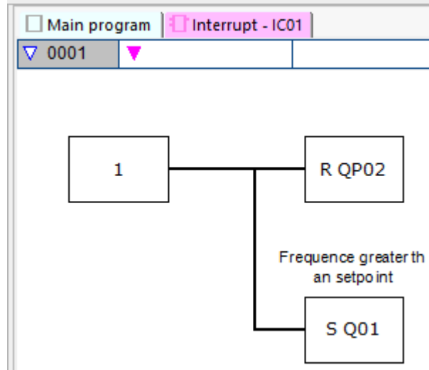
Abb. 216: easySoft 7 Interrupt-Programm Frequenzmessung
