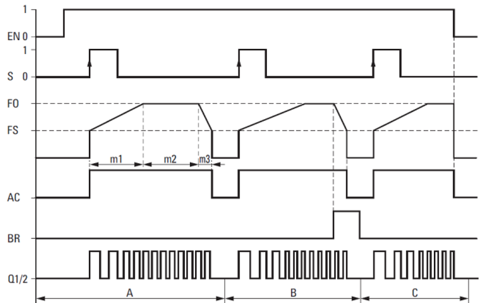
Abb. 168: Wirkdiagramm Impulsausgabe PO - mögliche Phasen des Normalbetriebs
