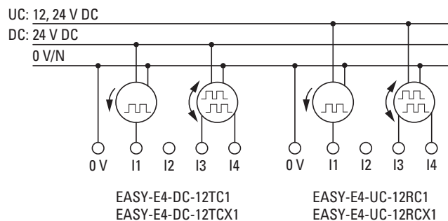
Abb. 17: digitale Zähler-Eingänge anschließen
