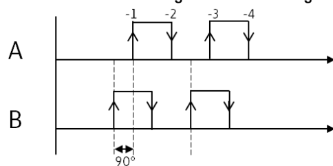
Abb. 148: Funktionsbaustein CI rückwärts zählend; QV=QV-4
