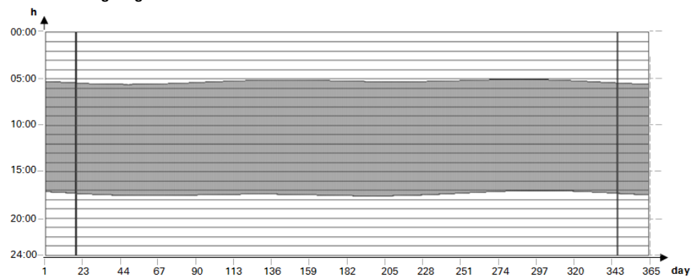
Abb. 137: Offset; O1=-2; O2=2; Q1=1 schaltet 2 Stunden vor Sonnenaufgang ein und 2 Stunden nach Sonnenuntergang aus
