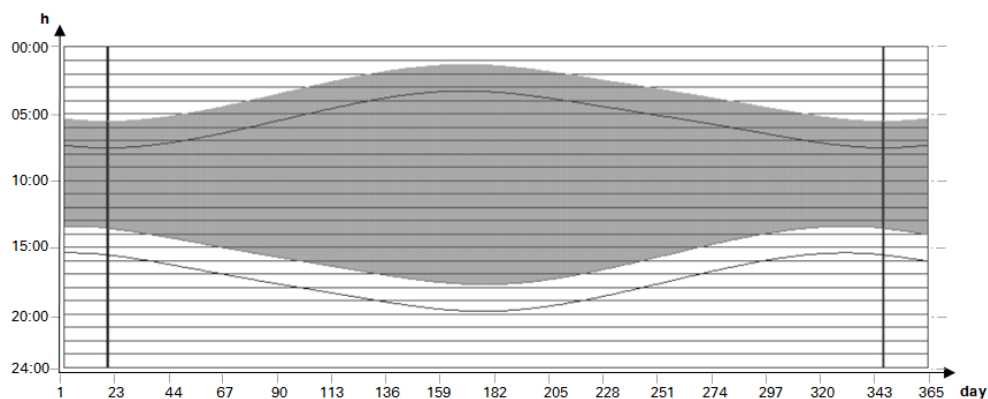
Abb. 141: Offset; O1=-2; O2=-2; Q1=1 schaltet 2 Stunden vor Sonnenaufgang ein und 2 Stunden vor Sonnenuntergang aus
