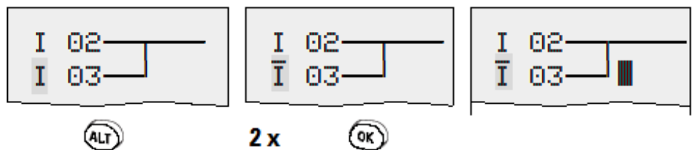
Abb. 83: Kontakt I 03 von Schließer zu Öffner ändern
