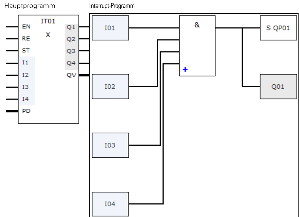
Abb. 220: Übergabe der Zustände von Ein- und Ausgängen zwischen Hauptprogramm und Interrupt-Programm
