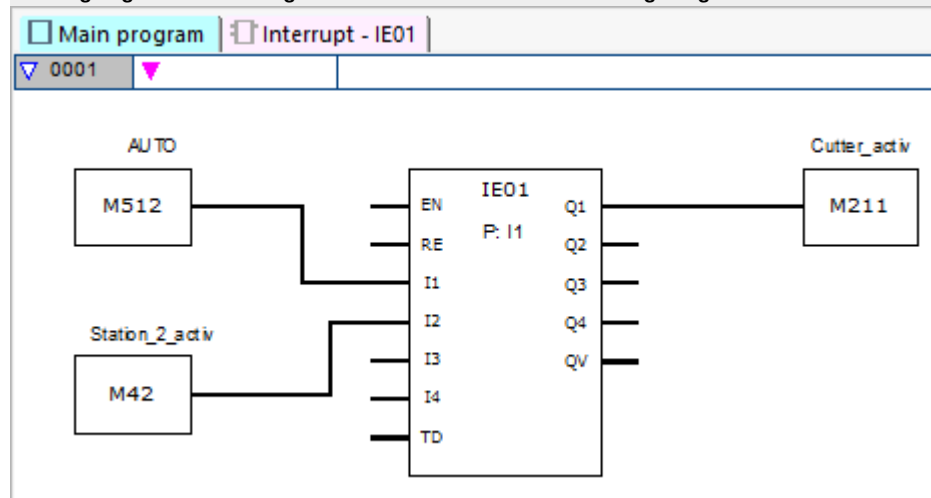
Abb. 218: easySoft 7 Hauptprogramm Flankengesteuert
