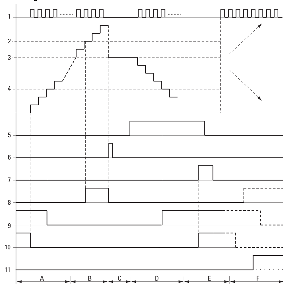
Abb. 144: Wirkdiagramm Zählrelais
