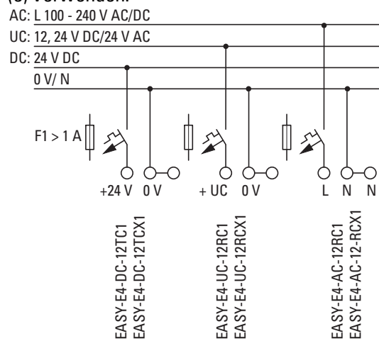
Abb. 13: Spannungsversorgung Basisgeräte anschließen
