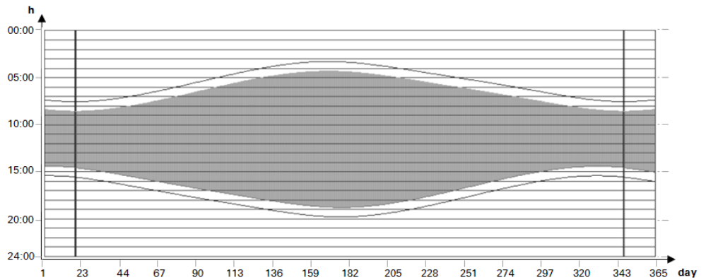
Abb. 139: Offset O1=1; O2= -1; Q1=1 schaltet 1 Stunde nach Sonnenaufgang ein und eine Stunde vor Sonnenuntergang aus
