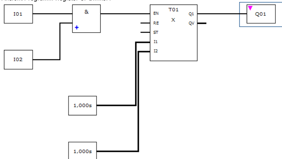
Abb. 226: Ansicht Programm Anwenderbaustein UF Blinker1
