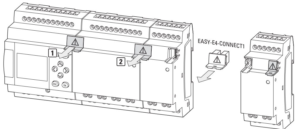
Abb. 10: benachbarte Verbindungsstecker entfernen
