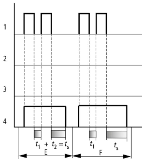
Abb. 121: Wirkdiagramm Zeitrelais rückfallverzögert
