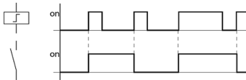
Abb. 75: Wirkdiagramm „Stromstoßrelais“
