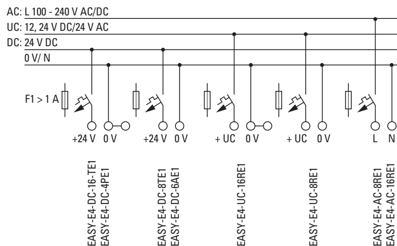
Abb. 14: Spannungsversorgung Erweiterungen anschließen
