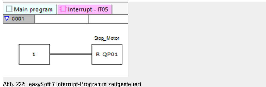
Abb. 222: easySoft 7 Interrupt-Programm zeitgesteuert
