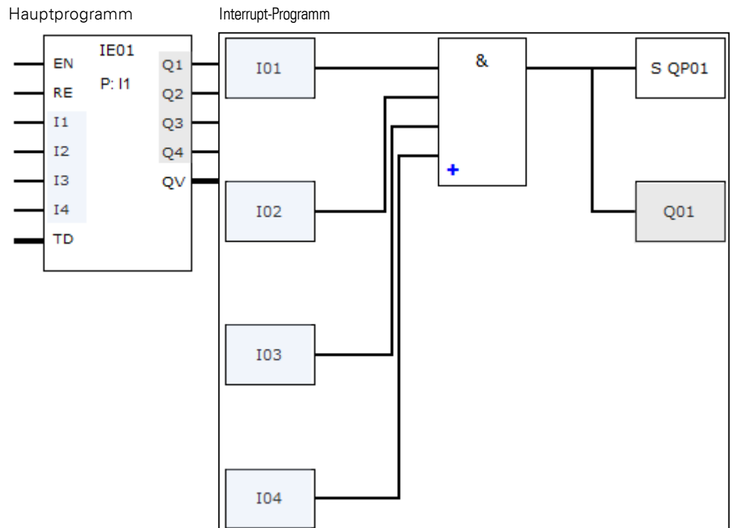
Abb. 217: Übergabe der Zustände von Ein- und Ausgängen zwischen Hauptprogramm und Interrupt-Programm
