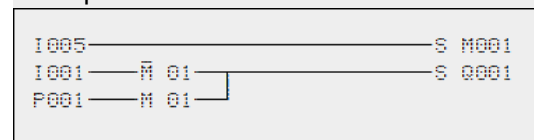
Abb. 92: I5 schaltet auf Cursor-Tasten um.
