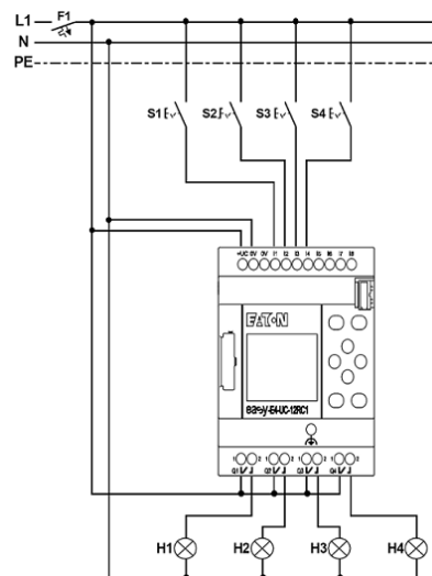
Abb. 299: Schaltplan easyE4 Lauflicht
