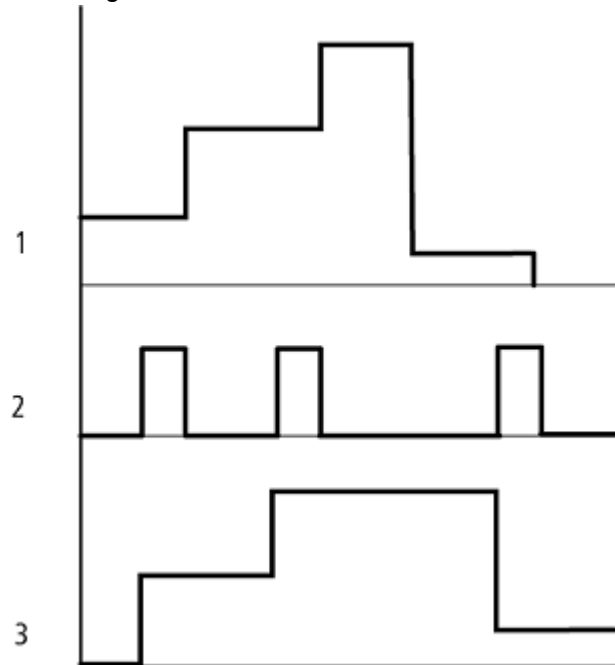
Abb. 182: Wirkdiagramm Datenbaustein
