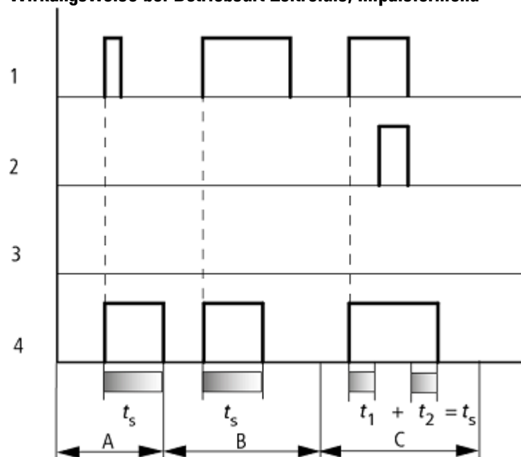
Abb. 123: Wirkdiagramm Zeitrelais, Impulsformend 1
