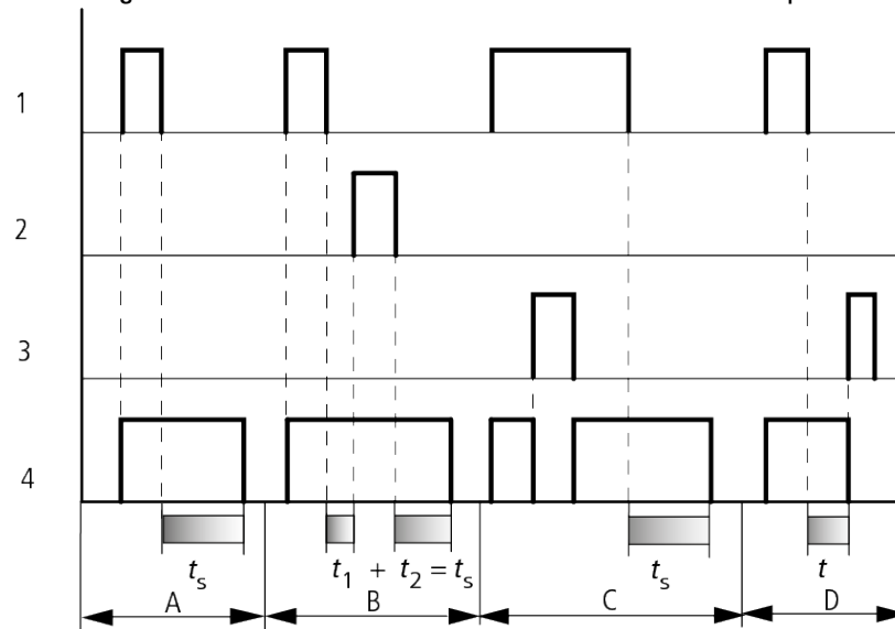
Abb. 120: Wirkdiagramm Zeitrelais rückfallverzögert
