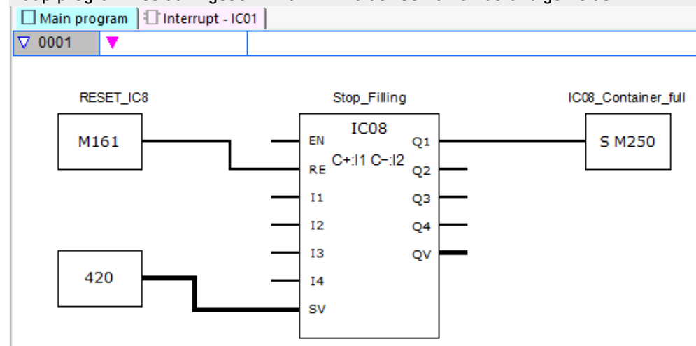
Abb. 211: easySoft 7 Hauptprogramm zwei Zählengänge
