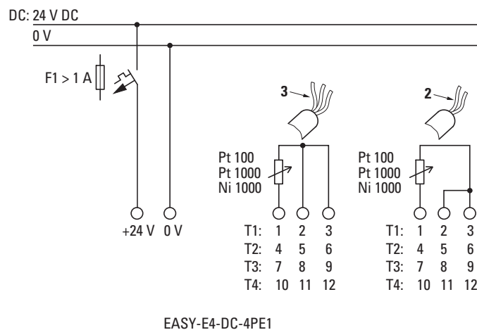
Abb. 26: analoge Eingänge EASY-E4-DC-4PE1 anschließen
