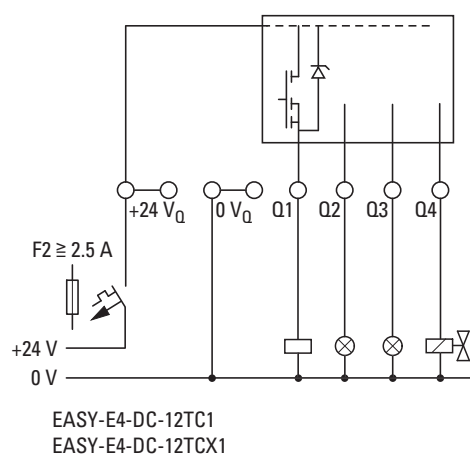
Abb. 20: Transistor-Ausgang Basisgerät anschließen
