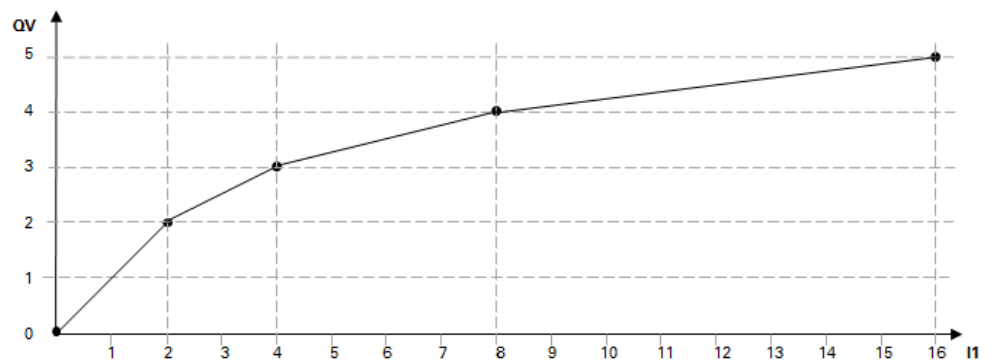
Abb. 160: Beispiel Kennlinie für Funktionsbaustein PM
