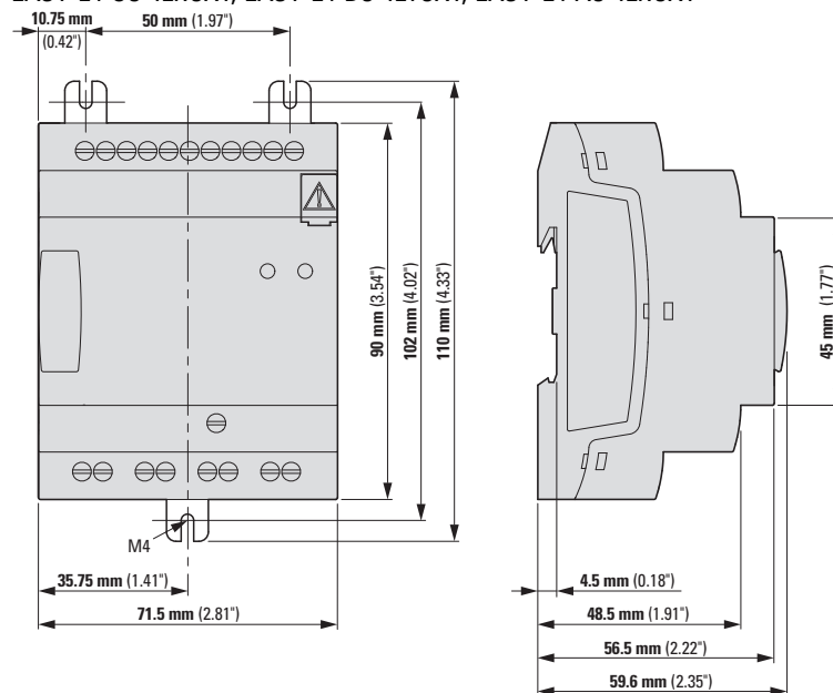
Abb. 295: Abmessungen in mm (Inch) Basisgeräte
