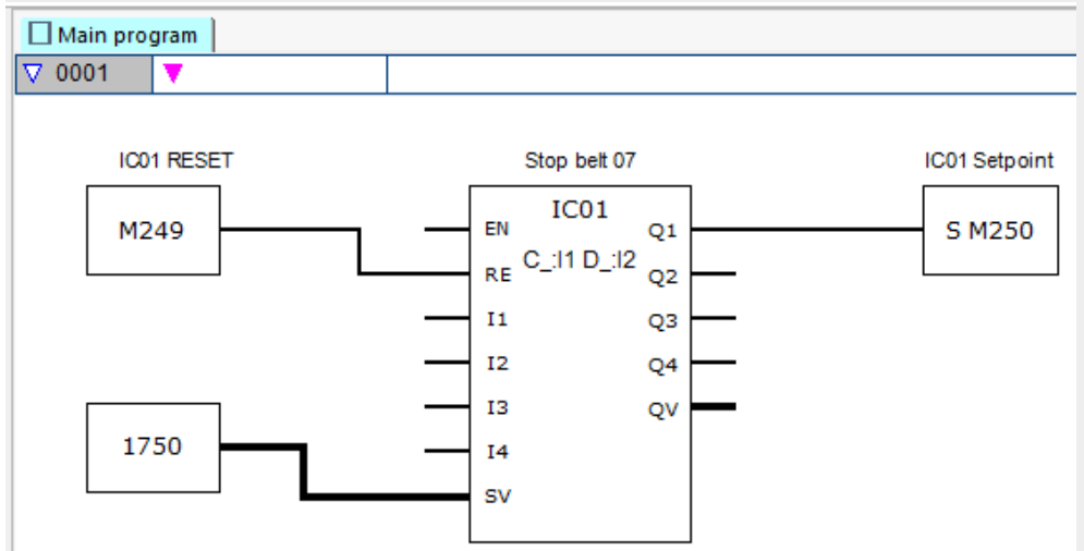
Abb. 209: easySoft 7 Hauptprogramm Impulszähler mit externer Richtung
