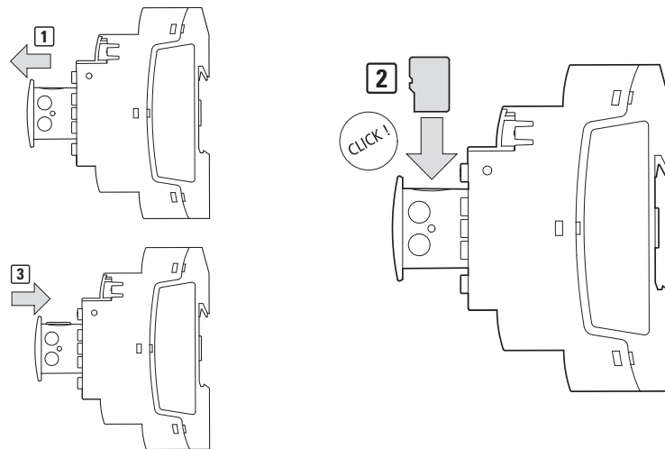
Abb. 30: Speicherkarte einsetzen
