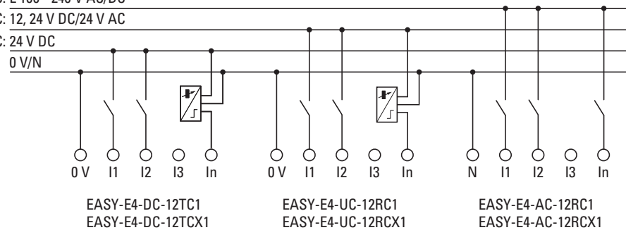
Abb. 15: digitale Eingänge Basisgeräte anschließen
