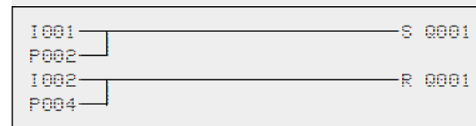
Abb. 91: Q1 über I1, I2, \wedge , oder \vee schalten
