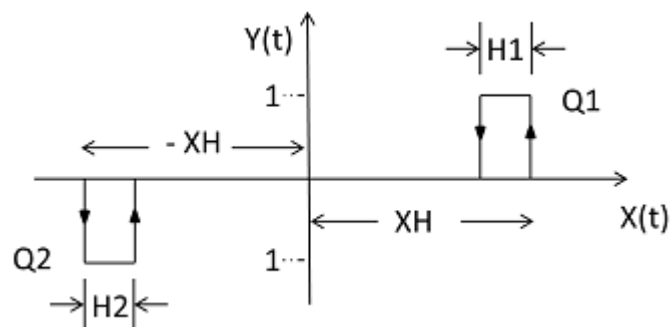
Abb. 173: Zeitdiagramm Dreipunktregler
