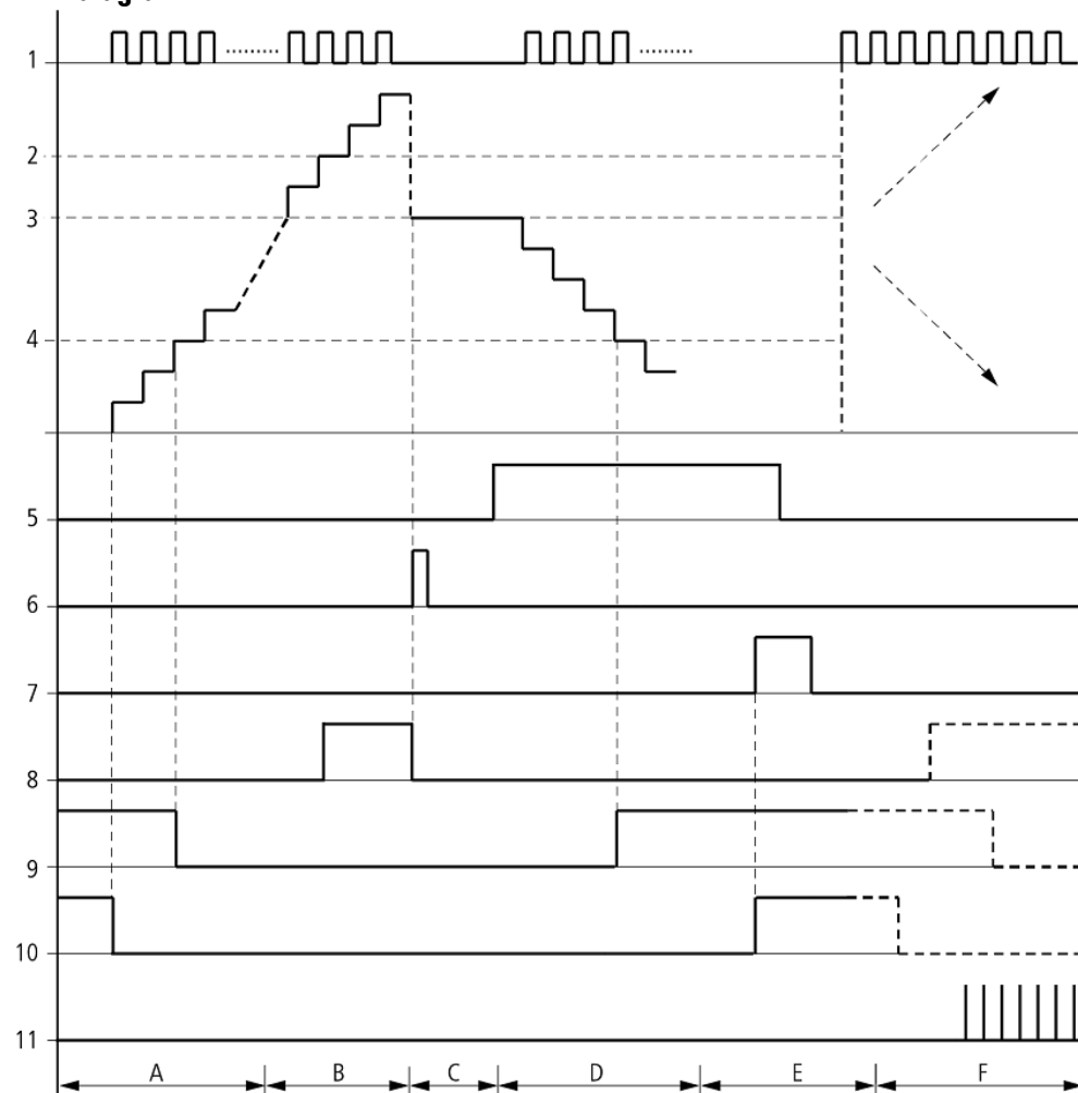
Abb. 149: Wirkdiagramm Schneller Inkrementalwertzähler
