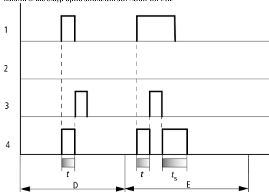
Abb. 124: Wirkdiagramm Zeitrelais, Impulsformend 2
