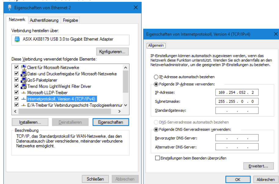
Abb. 72: Ethernet-Verbindung am PC
