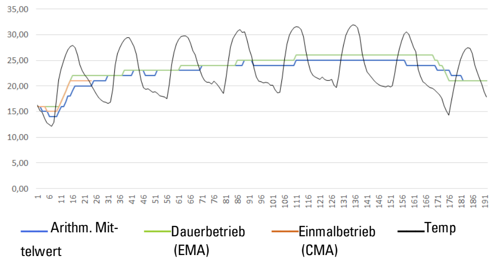
Abb. 154: Beispielkennlinie Temperaturmessung stündlich, über 7 Tage
