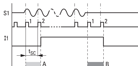
Abb. 261: Schaltverhalten AC-Eingangssignal bei aktivierter I-Entprellung
